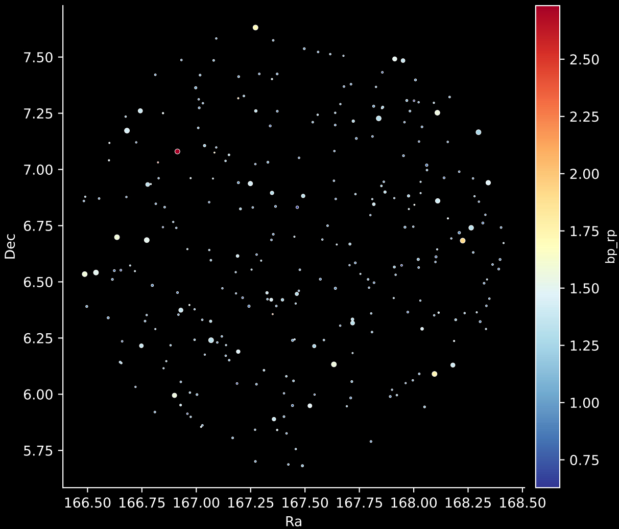
GALAH DR4 Field: [1239] Stars: 290
