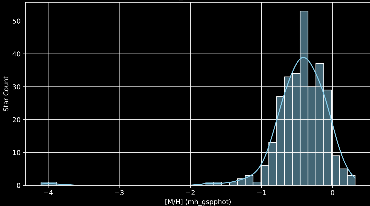
GALAH DR4 Field: [1239] [M/H] (mh_gspphot) (n= 290)
