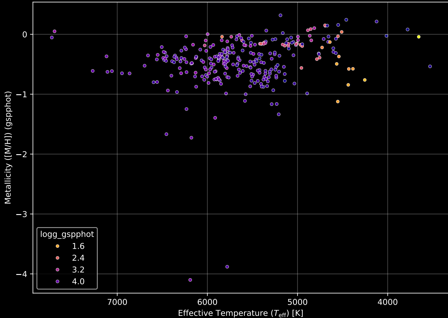
GALAH DR4 Field: [1239] Stellar Population Parameters (n= 290)
