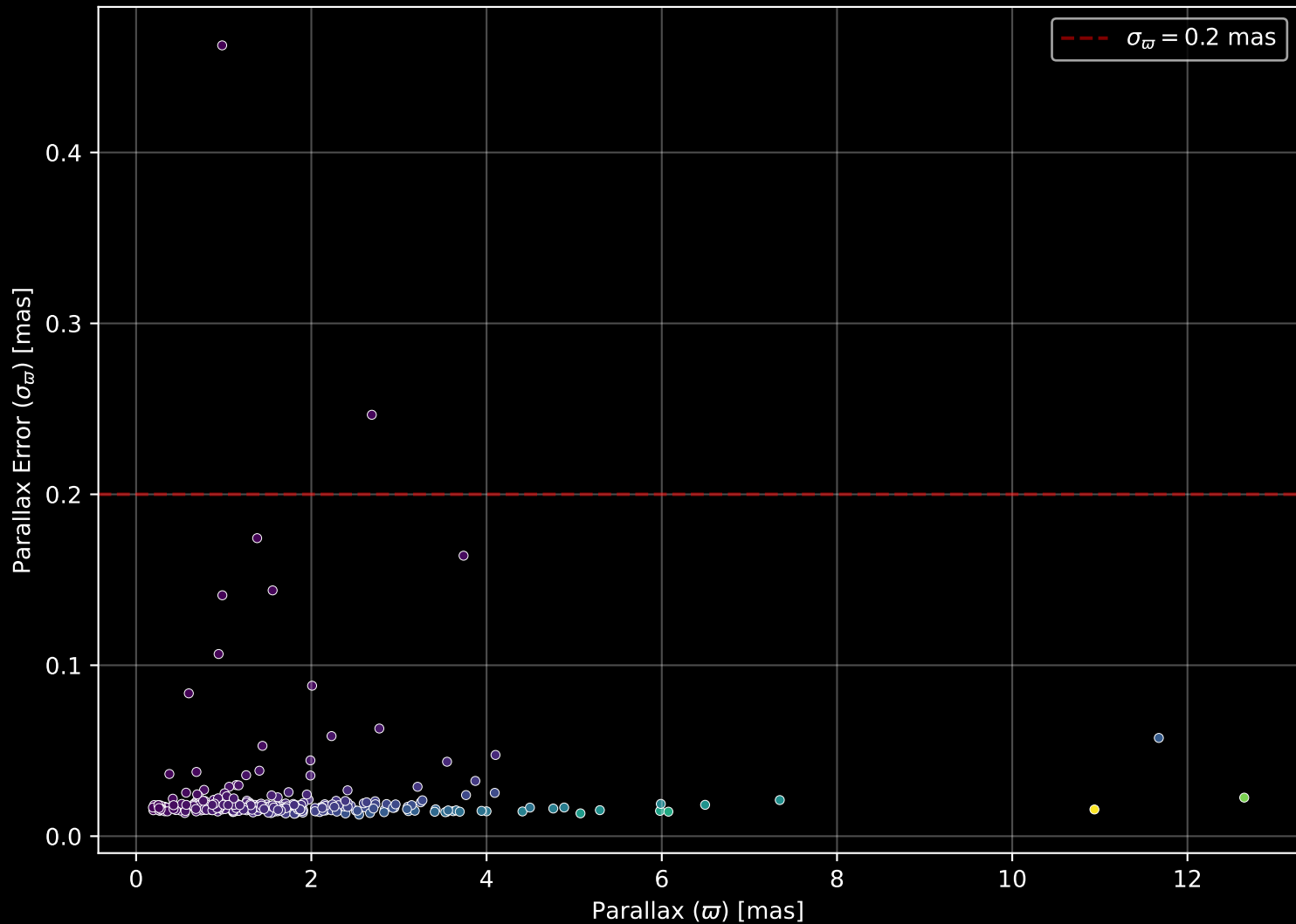
GALAH DR4 Field: [1239] Parallax Quality (n= 290)
